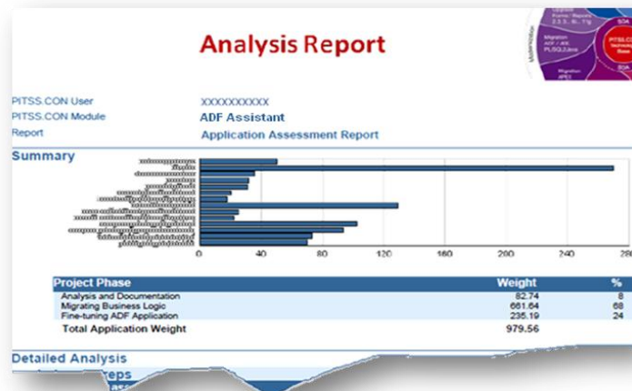
Abbildung 7: PITSS.CON Anwendungsanalyse-Bericht
