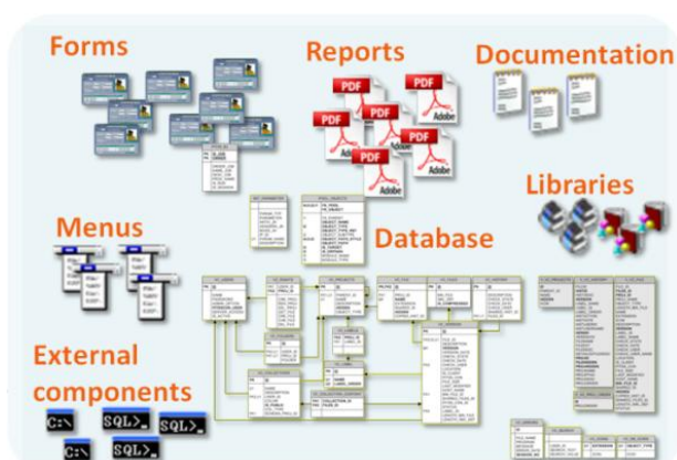
Abbildung 3: Typische Forms-Anwendungskomponenten
